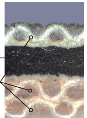
Newly developed low stretch 3-layer carcass for outstanding stability / Neu entwickelte Karkasse für eine hervorragende Stabilität
